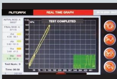
Resultados del ensayo de módulo elástico
